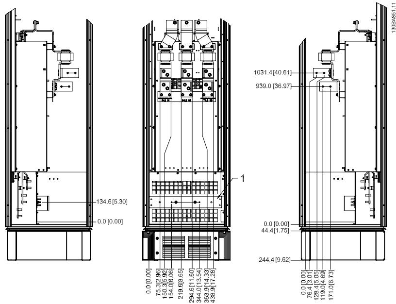
Рисунок 3.22: Расположение клемм - шкаф дополнительных устройств (вид слева, спереди и справа)
