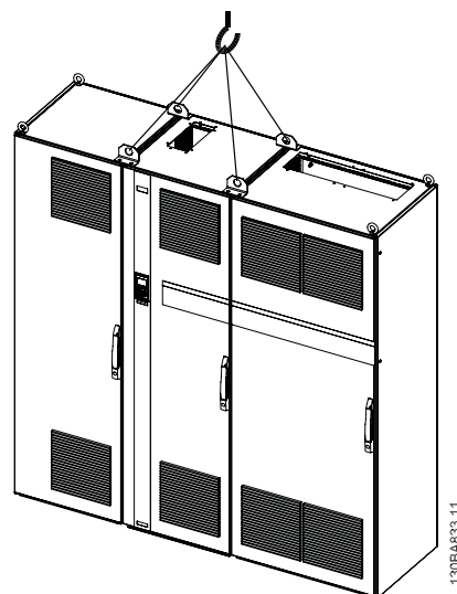
Рисунок 3.6: Рекомендуемый метод подъема, размер корпуса F3.
