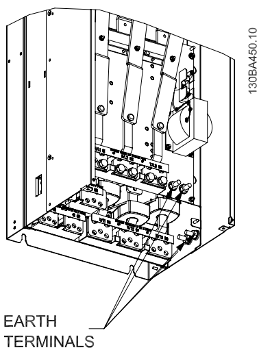
Рисунок 3.40: Расположение клемм заземления IP00, размеры корпуса D
