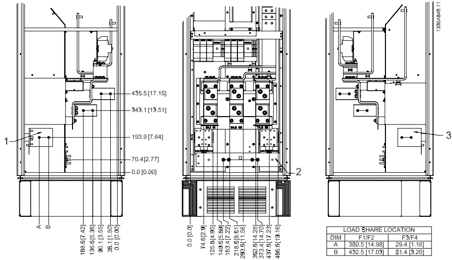
Рисунок 3.21: Расположение клемм - выпрямитель (вид слева, спереди и справа)
