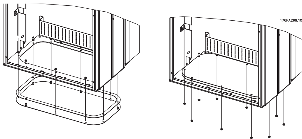
Рисунок 3.26: Монтаж нижней платы, Размер корпуса E1.
