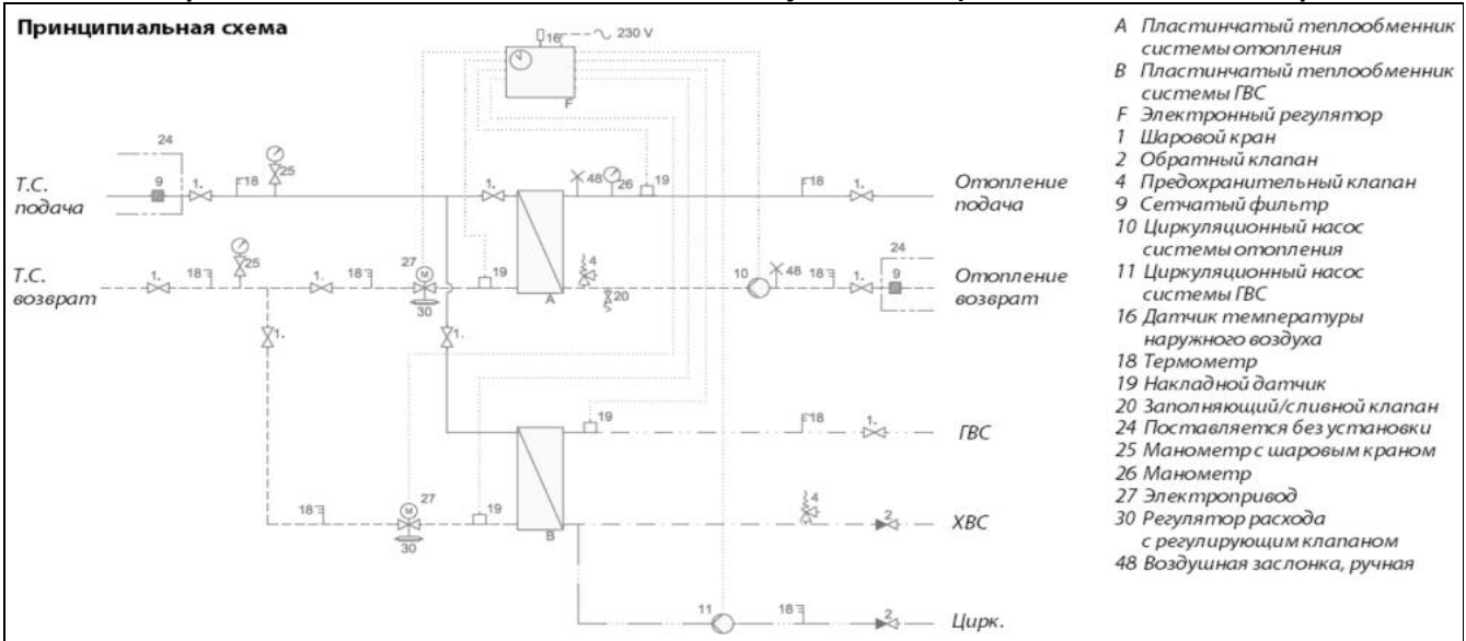
Рис. 10. Принципиальная схема малого теплового пункта модификации Termix VVX Compact 28-40
