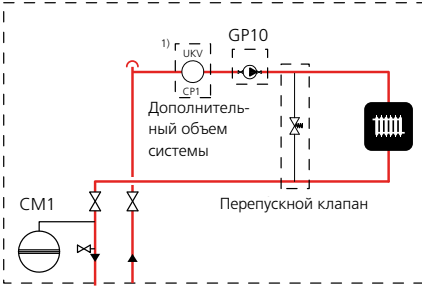
Радиаторная система
