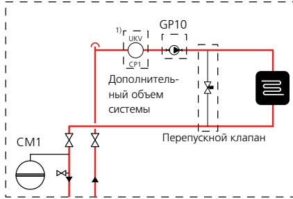
Система отопления «теплый пол»
