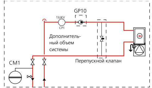
Система вентиляторных конвекторов
