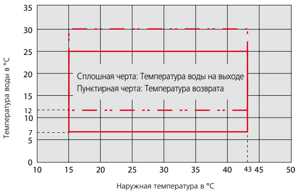
Рабочий диапазон компрессора - Охлаждение
