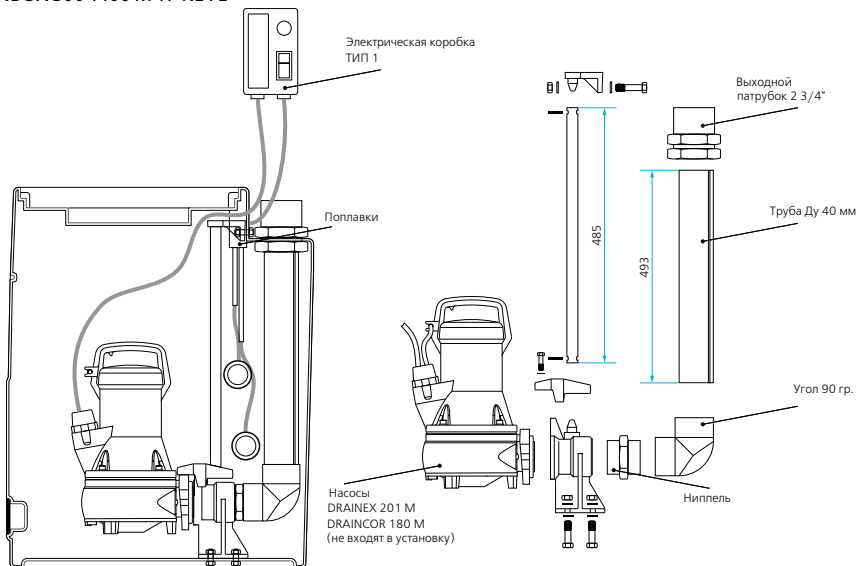
Комплект обвязки для установки DRAINBOX 300 1400 M TP KE FL
