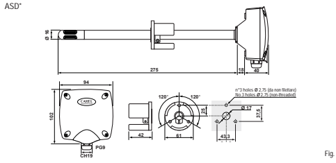
Dimens. sonde da condotta (ASD*) e da ambiente tecnico (ASP*) / Duct probes (ASD*) and general purpose (ASP*) dimens.
