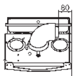
Забор воздуха/отвод продуктов сгорания по коаксиальным трубам
