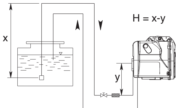
Tubo doble de la parte superior del depósito
