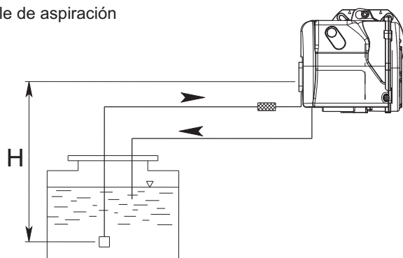
Tubo doble de aspiración
