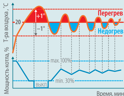
► Работа пропорционального (модулирующего) термостата при поддержании 20°C
