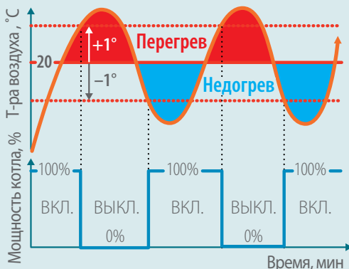
► Работа 2-х позиционного (ВКЛ./ВЫКЛ.) термостата при поддержании 20°C
