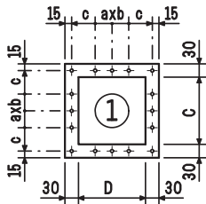
Refoulement ventilateur
