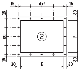
Aspiration centrale
