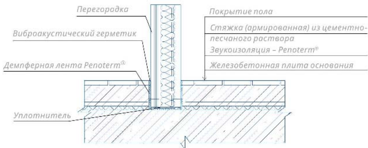
Рис. 1.2. Узел сопряжения пола с перегородкой
