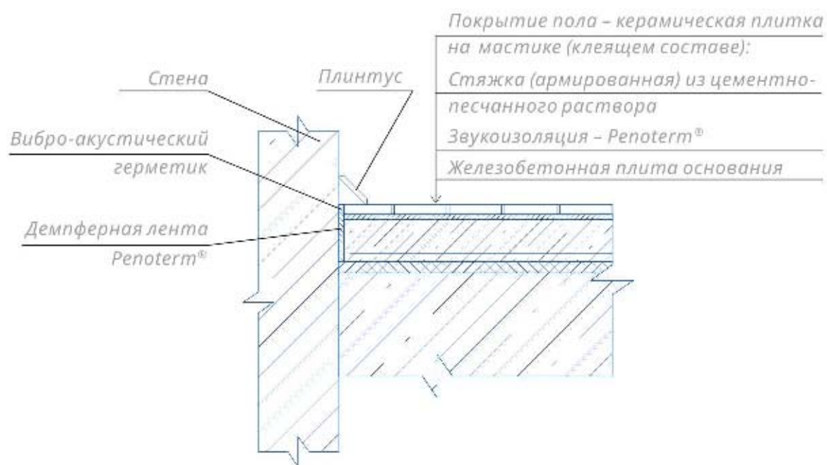
Рис. 1.6. Узел примыкания плиточных полов к стене
