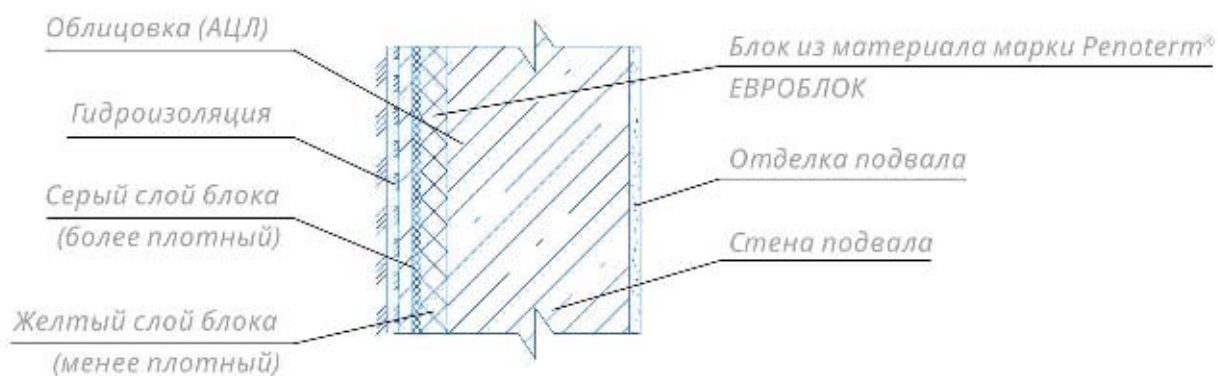
Рис. 3.5. Состав стены подвала с наружным утеплением
