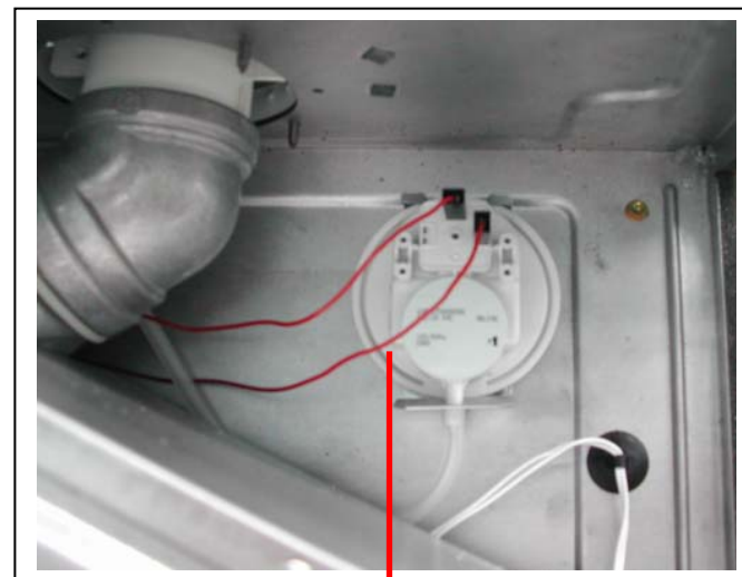
Переключатель давления воздуха
