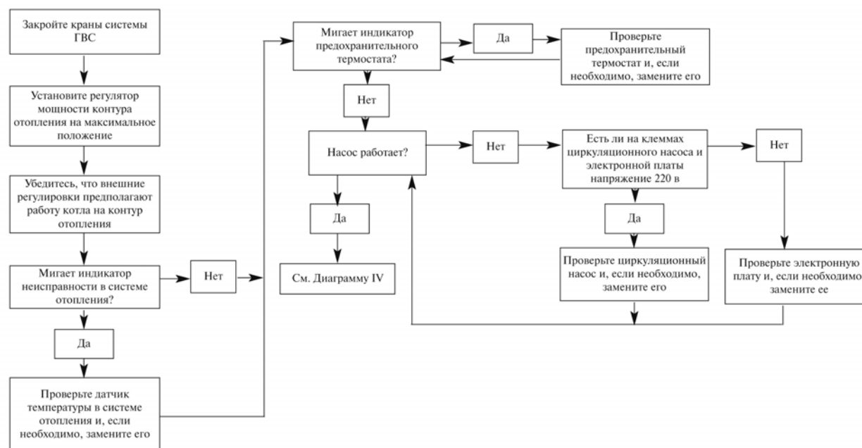
Диаграмма III Тестирование системы отопления
