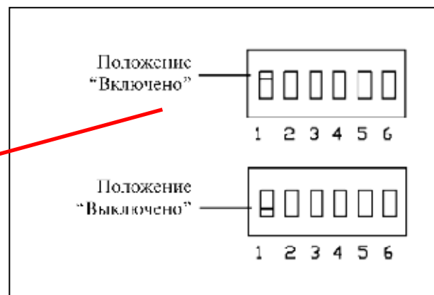
Переключки
