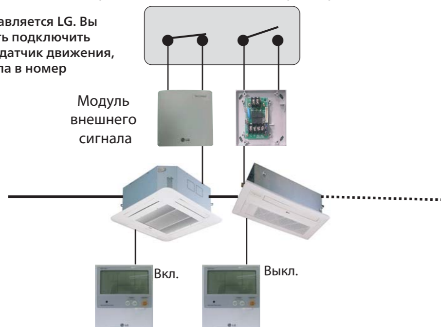
Переключатель внешних контроллеров
