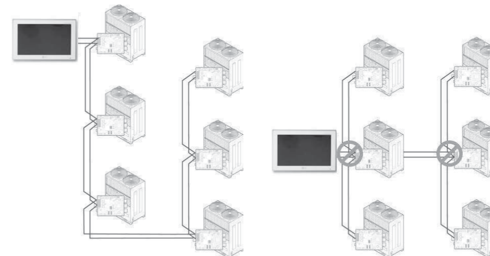
<Правильно: соединение RS485 BUS>>
