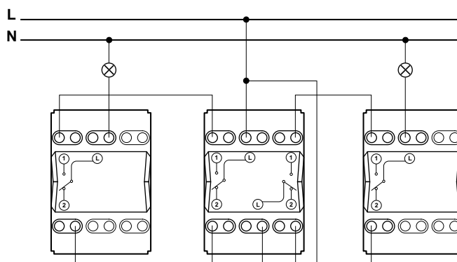
2 выключателя на два направления + 1 двухклавишный выключатель на два направления, работающий с разными нагрузками
