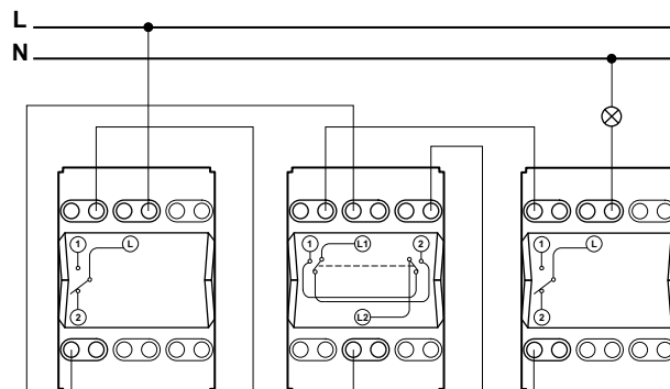
2 выключателя на два направления + 1 промежуточный выключатель
