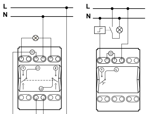
Двухполюсный выключатель с лампами подсветки
