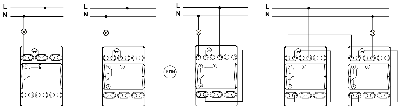
Выключатель с лампами подсветки
