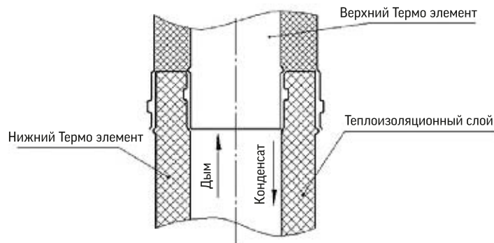
Рис.1 Схема соединения элементов дымохода
