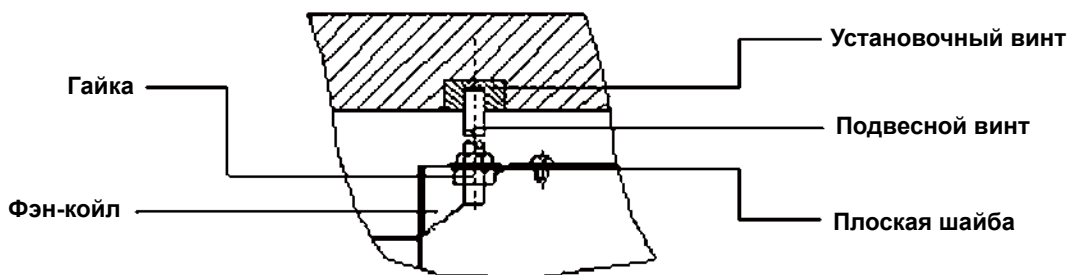
Рис.3 - Деталь А
