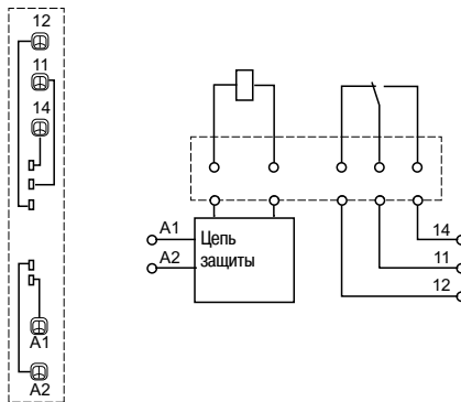
RSL ZR●● с пружинными клеммами
