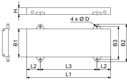
Рис. 87 Рама-основание EN/ISO с 4 установочными отверстиями
