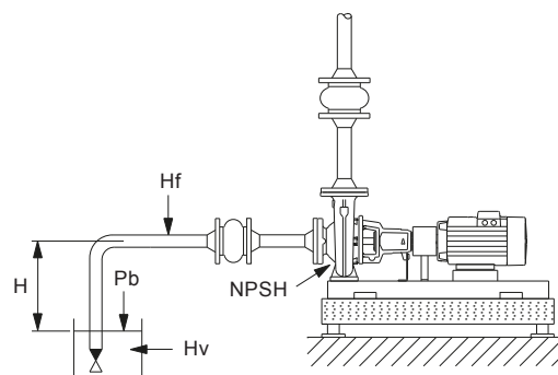
Рис. 47 Высота всасывания воды при положительном значении H_{всас}
