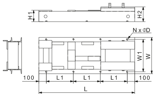
Рис. 93 С-образная рама-основание с 8 установочными отверстиями
