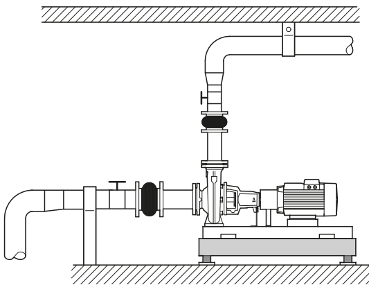
Рис. 56 Монтаж трубопровода
