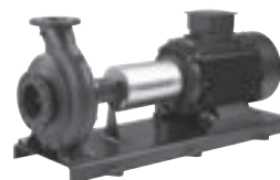
Рис. 2 Консольный насос (NKG)
