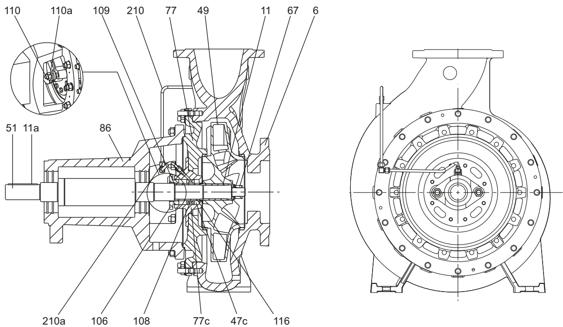
Рис. 17 Чертеж в разрезе, сальник с разъемной крышкой
