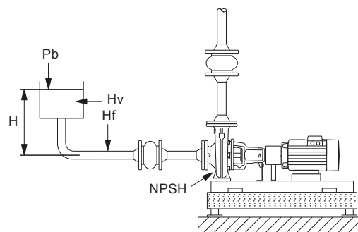
Рис. 48 Высота всасывания воды при отрицательном значении H_{всас}
