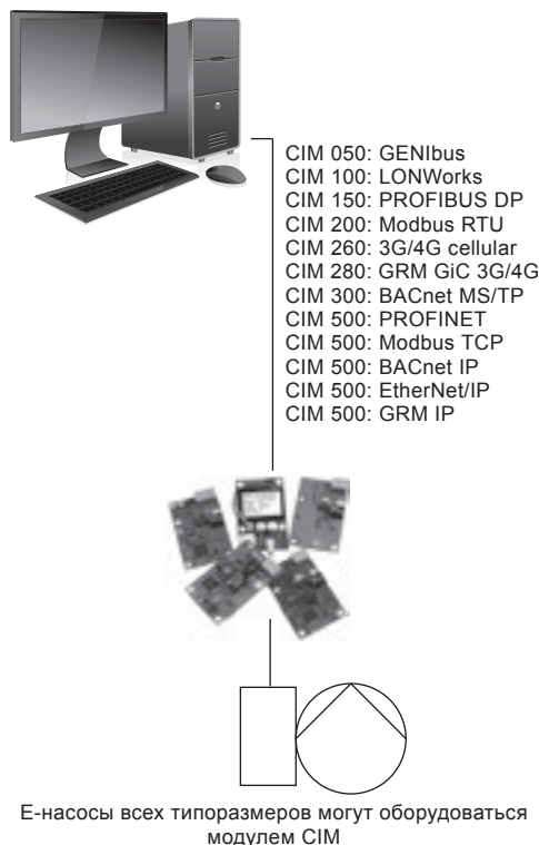
Рис. 71 Структура центральной системы управления внутримодовыми коммуникациями
