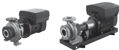
Рис. 61 Насосы NBGE, NKGE без датчиков с завода
