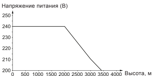
Рис. 41 Напряжение питания для однофазного электродвигателя в зависимости от высоты над уровнем моря
