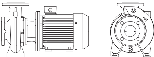
Рис. 20 Исполнение С
