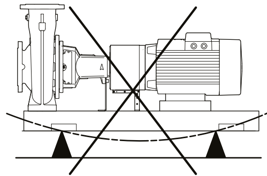
Рис. 51 Неправильная установка
