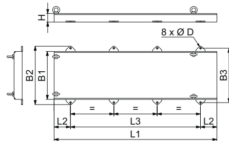
Рис. 90 Рама-основание EN/ISO с 8 установочными отверстиями
