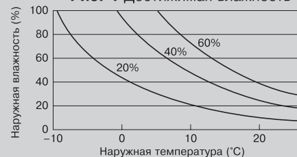
Рис. 1 Достижимая влажность
