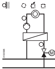
Контур отопления с подключением к районному теплоснабжению
