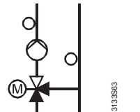
Первичный контроллер и смешивательный клапан
