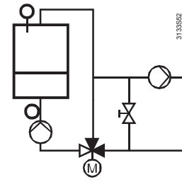
Поддерживаемая обратка бойлера при помощи смешивающего клапана
