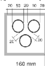
Минимальные внутренние размеры камеры для прохода трех дымоходов, диаметр 50 мм
