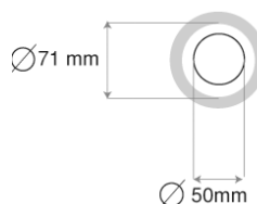
Минимальные внутренние размеры камеры для прохода 1 дымохода, диаметр 50 мм
