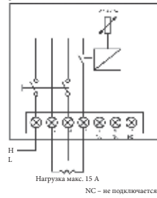
Devireg™ 531
