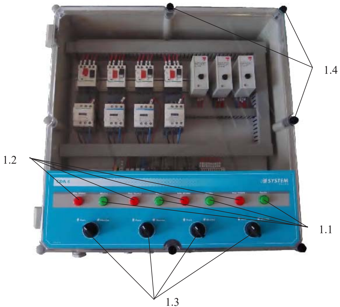
Рисунок 1 – Шкаф управления CDA. Общий вид
