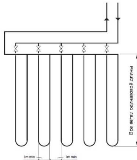
Многовитковый коллектор
