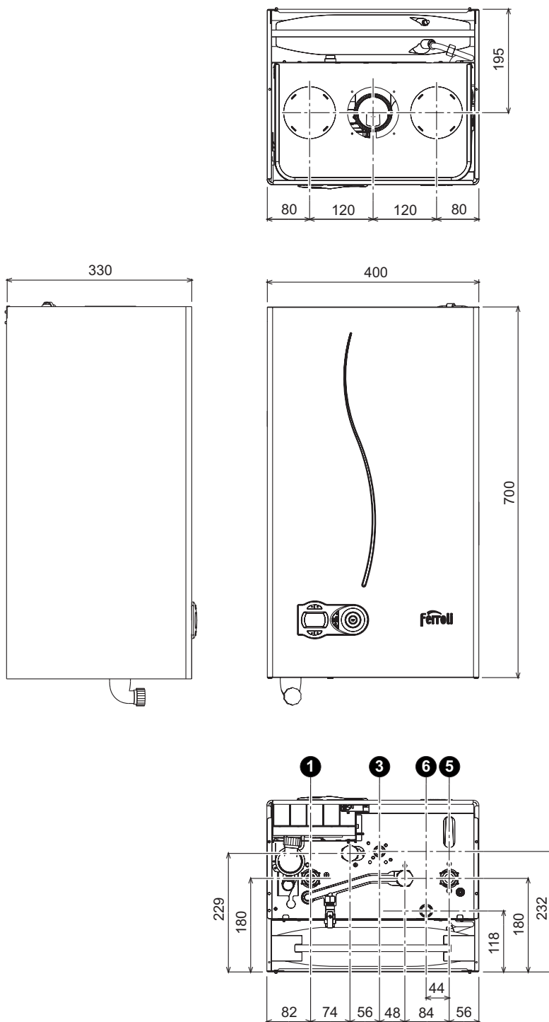
рис. 31 - Габаритные размеры и присоединения
