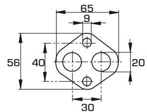
Фланец
