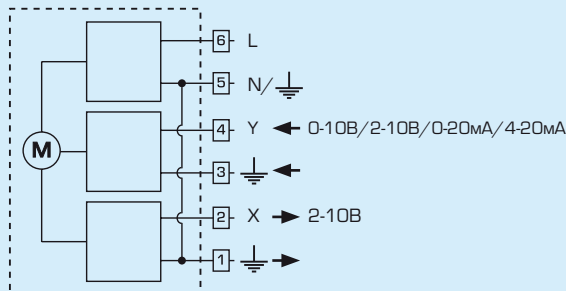
Привод серии АРА639
