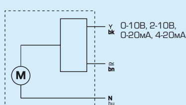
Привод серии АРА659
