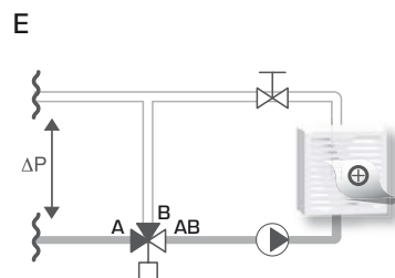
Установка совместно с местным циркуляционным насосом в контуре
