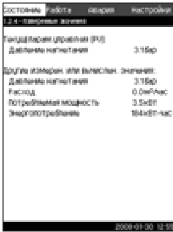
Рис. 14 Измеренные значения
