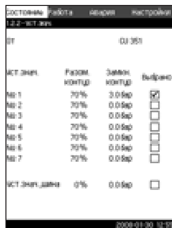
Рис. 12 Установленное значение
