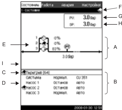
Рис. 8 Состояние
