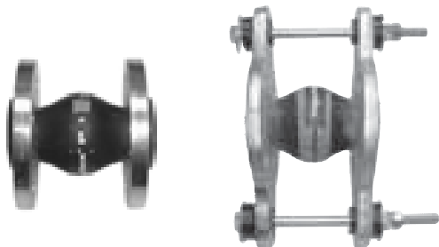
Рис. 5 Вибровставки с резиновыми прокладками без ограничительных стяжек и с ними
