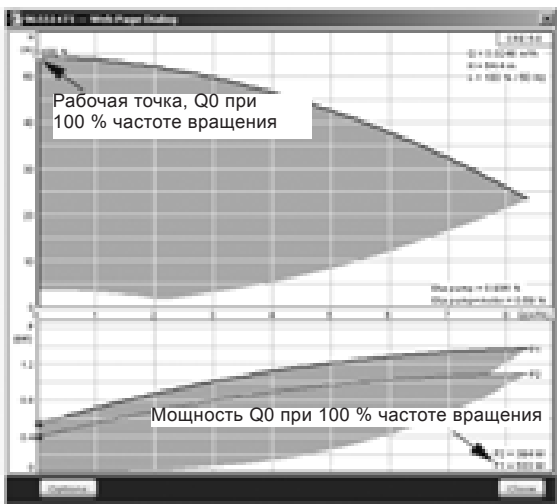
Рис. 82 Показание мощности Q0 при 100 % частоте вращения (WebCAPS)
