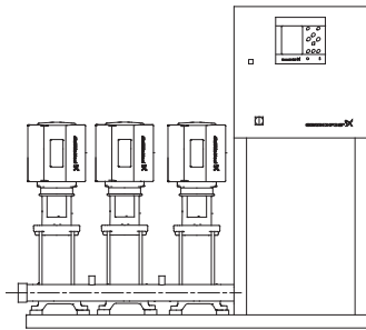
Рис. 20 Установка, регулируемая встроенным ПИ контроллером (замкнутый контур)
