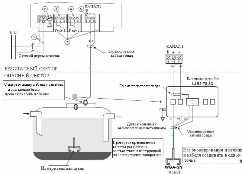
Рисунок 3. Установка WGA 04
