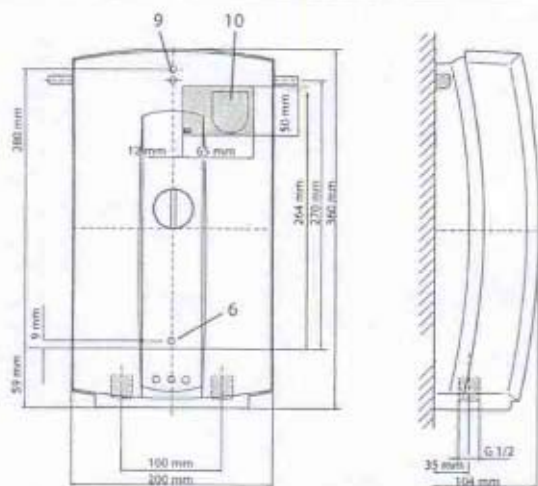
Расположение прибора
