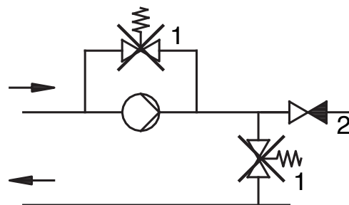
Рис. 3. Использование в трубопроводах перепускного и обратного клапанов
