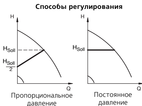
Рис. 9. Способы регулирования насосов UPE серии 2000
