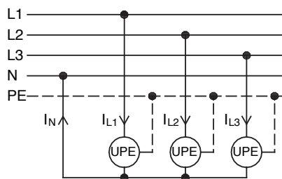
Рис. 5. Подключение трех насосов UPE к трем фазам
