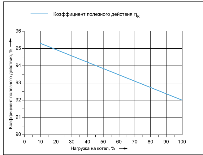
Диаграмма: Коэффициент полезного действия в зависимости от нагрузки на котел
