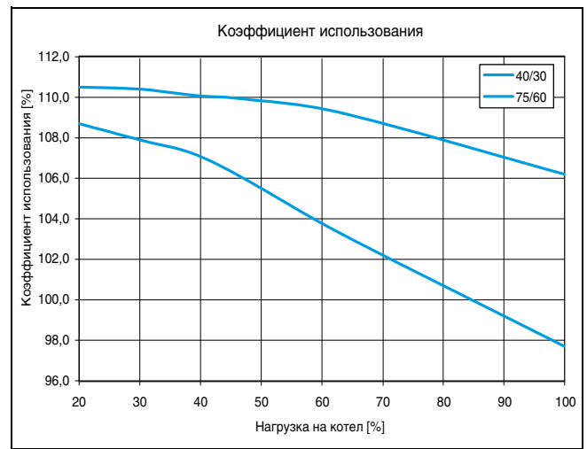
Кэффициент использования в зависимости от средней температуры котловой воды
