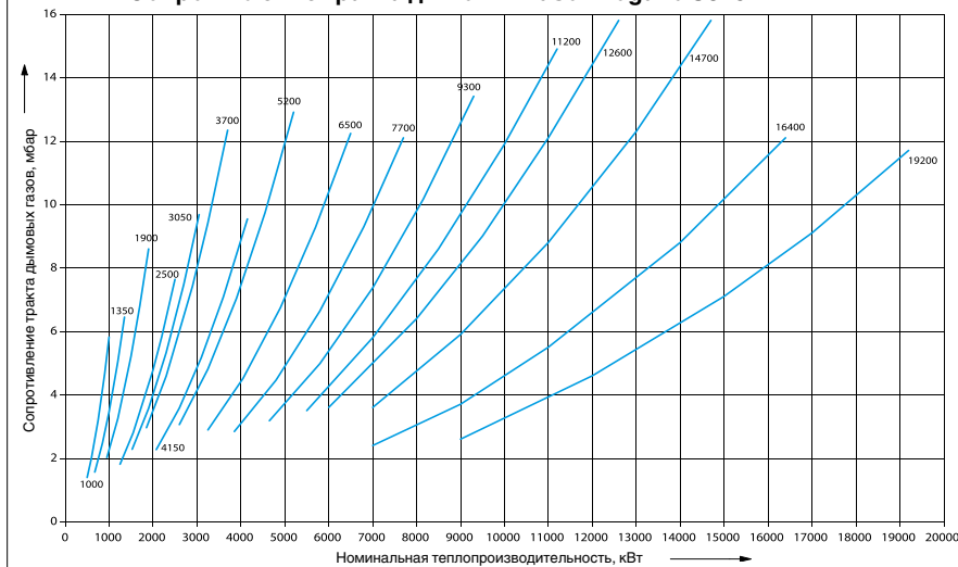
Объемная нагрузка на камеру сгорания Logano S815L LN
