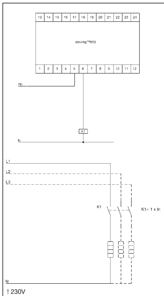
Рис. С. Грунт, 1-3 фазы, 1-3 кабеля на 230В
