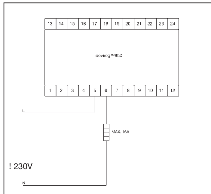
Рис.Г. Грунт, прямое подключение кабеля
