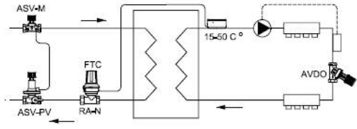
Радиаторная система отопления или обогрева пола с теплообменником
