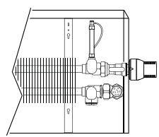
Вентиль Jaga - подсоединение к стене
