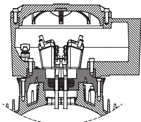
Типоразмеры электродвигателей 280–315
