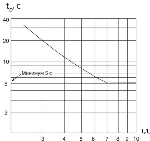
Рис. 2. Мин. значение времени t_E в зависимости от I_A/I_N согласно EN 50019
