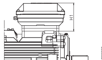
Типоразмеры электродвигателей 355–400
