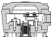
Типоразмеры электродвигателей 80–132
