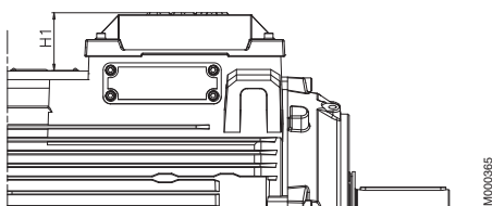
Типоразмеры электродвигателей 280–315
