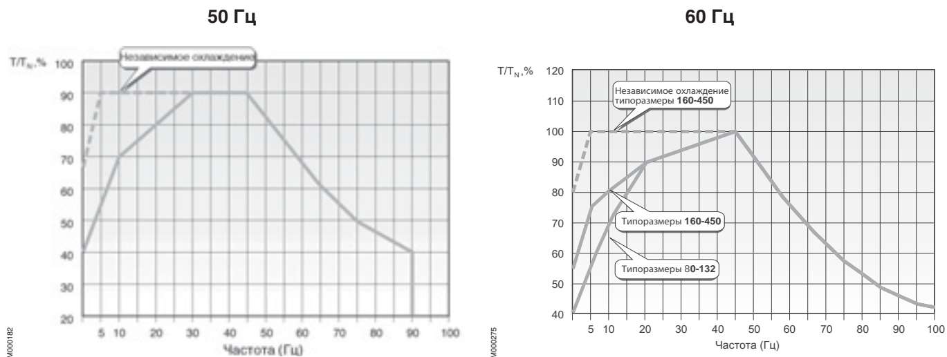
Рис. 3. Искробезопасные электродвигатели Ex nA, электродвигатели с защитой от воспламенения горючей пыли (DIP/Ex tD T 150 °C), с чугунной (тип M3GP) и алюминиевой станиной, номинальная частота электродвигателя 50/60 Гц
