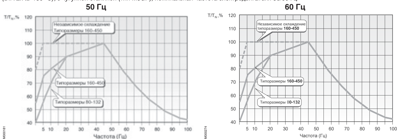
Рис. 3. Искробезопасные электродвигатели Ex nA, электродвигатели с защитой от воспламенения горючей пыли (DIP/Ex tD T 150 °C), с чугунной (тип M3GP) и алюминиевой станиной, номинальная частота электродвигателя 50/60 Гц
