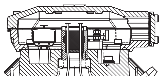
Типоразмеры электродвигателей 80–132
