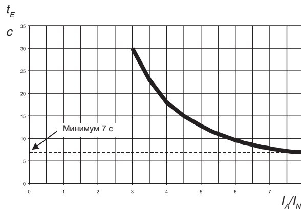
Рис. 3. Мин. значение времени t_E в зависимости от I_A/I_N согласно VIK
