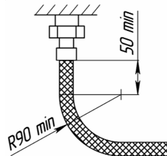
Рисунок 7. Требования к изгибам гибких шлангов
