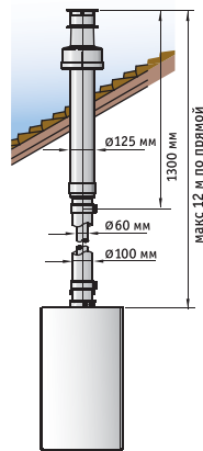
Вертикальный коаксиальный дымоход
