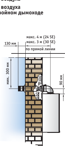
Коаксиальный горизонтальный дымоход
