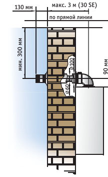
Коаксиальный горизонтальный дымоход
