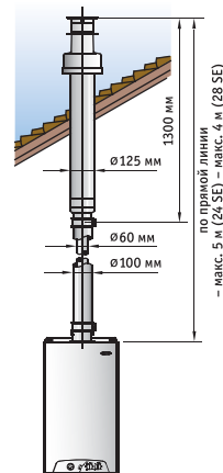
Вертикальный коаксиальный дымоход
