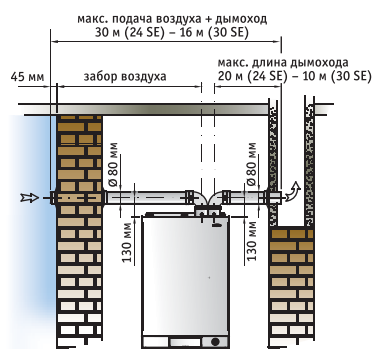
Двойной горизонтальный дымоход
