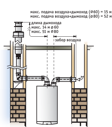
Двойной дымоход
