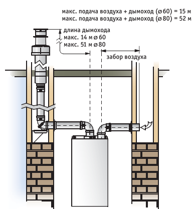
Двойной дымоход
