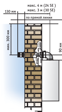
Коаксиальный горизонтальный дымоход
