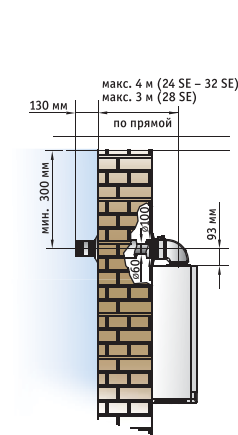
Коаксиальный горизонтальный дымоход
