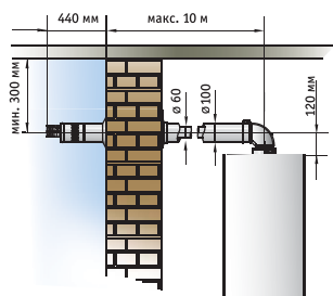
Коаксиальный дымоход
