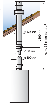
Вертикальный коаксиальный дымоход
