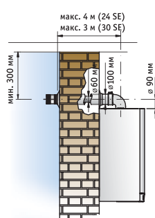
Коаксиальный горизонтальный дымоход
