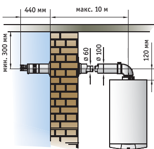
Коаксиальный дымоход
