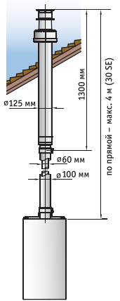
Вертикальный коаксиальный дымоход
