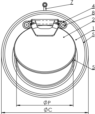
DN 300-400 Без пружины, только вертикальная установка
