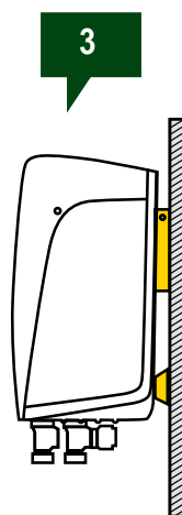
▶ НАСТЕННАЯ УСТАНОВКА с e.sywall
