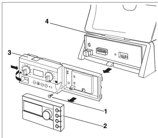
Рис. 3 Демонтаж RC30/BC10 (принципиальная схема)
