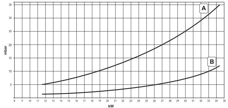
fig. 34 - DIVAtop 60 F 32
