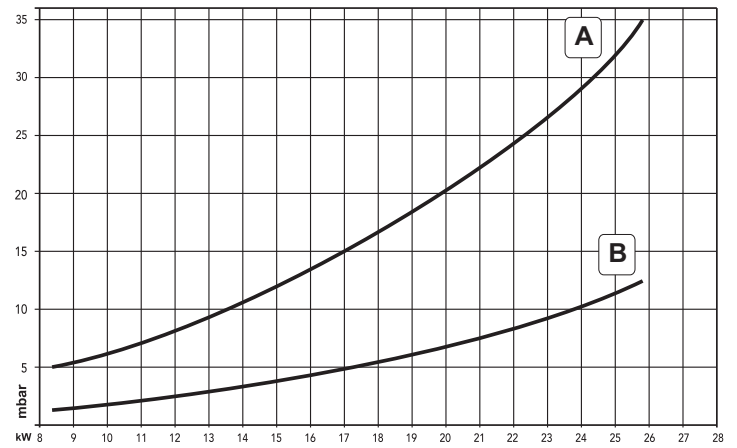
fig. 33 - DIVAtop 60 F 24
