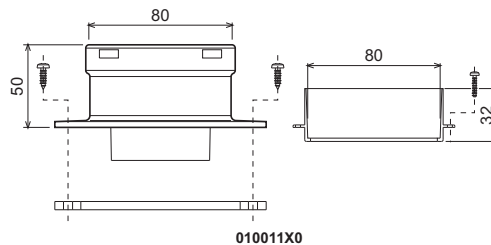
рис. 24 - Соединительный элемент для раздельных труб
