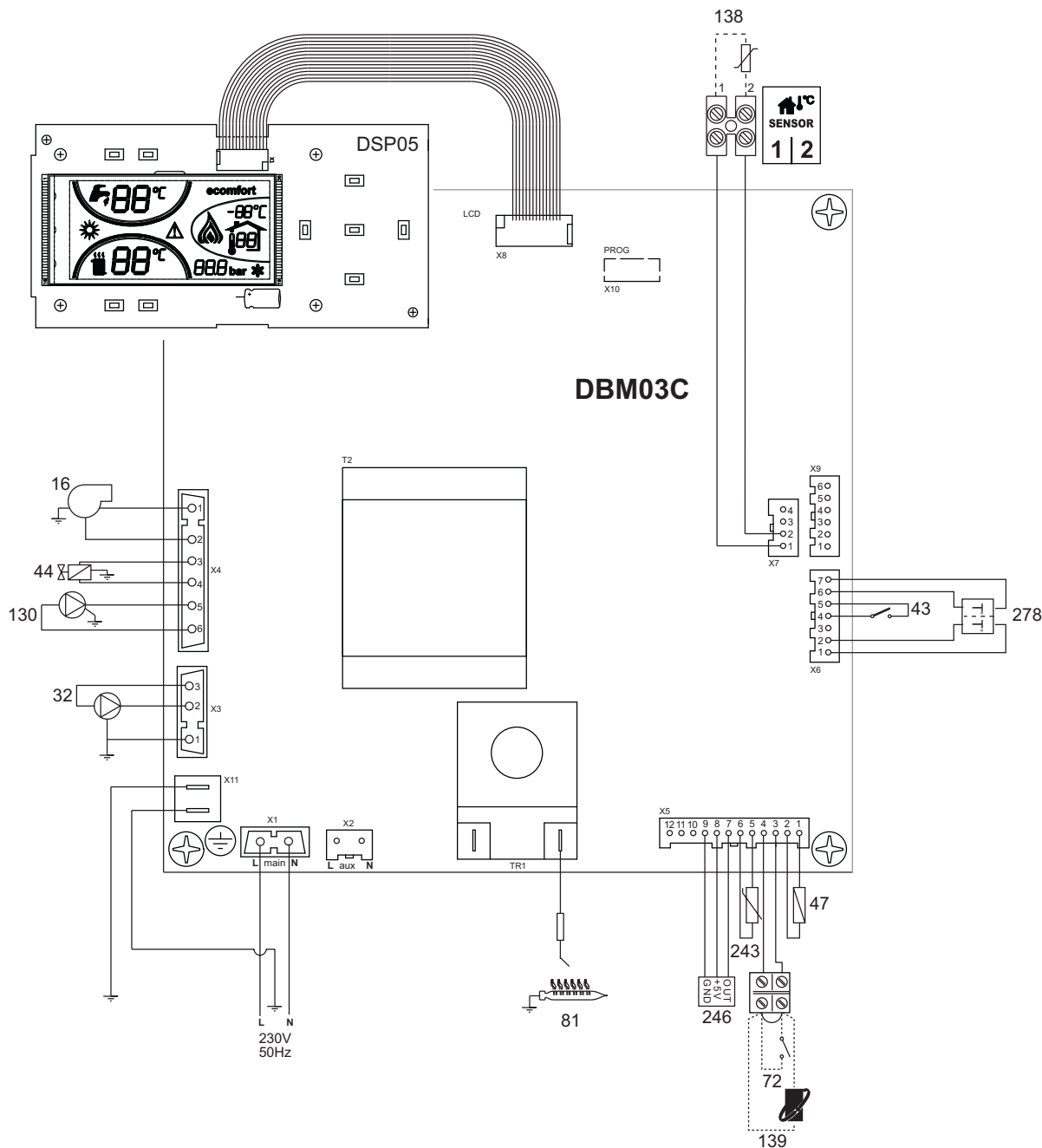
рис. 37 - Электрическая схема
