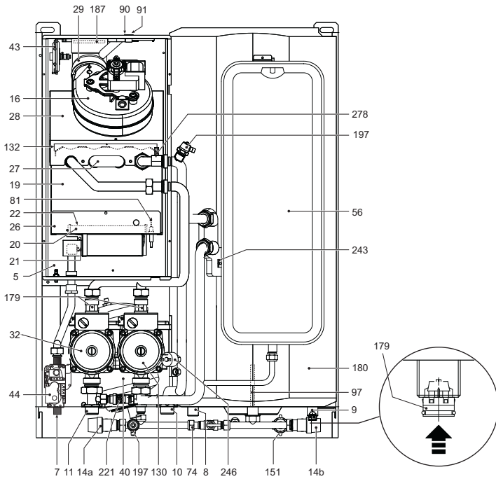
рис. 31 - Общий вид
