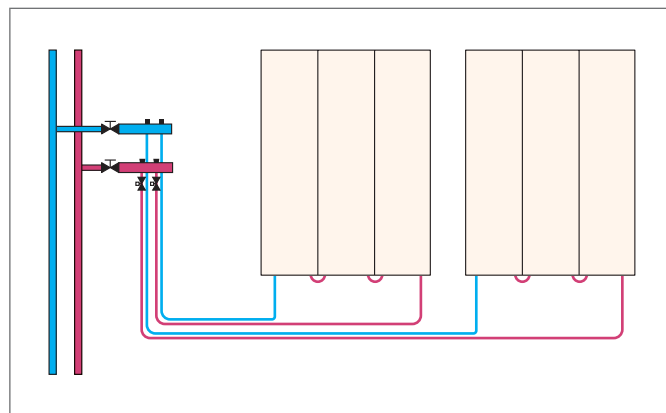
Рис. 4-41 Последовательное соединение нескольких панелей при коллекторной разводке
