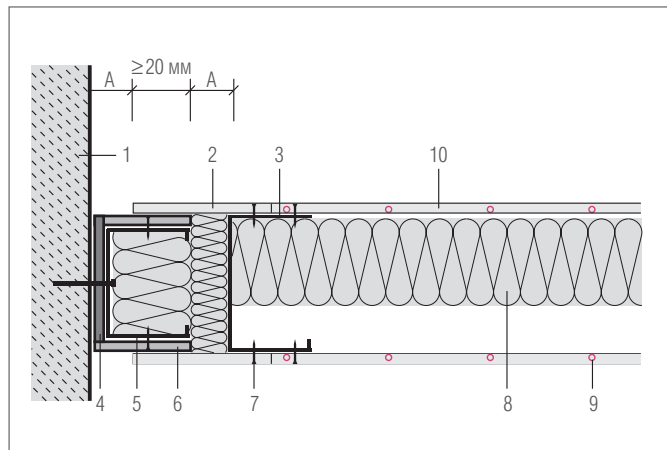
Рис. 4-36 Скользяще примыкание стен
