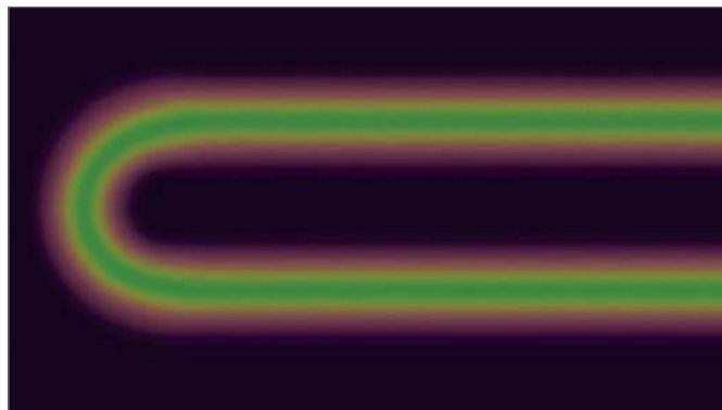
Рис. 4-28 Поиск мест прокладки труб, по которым движется теплоноситель
