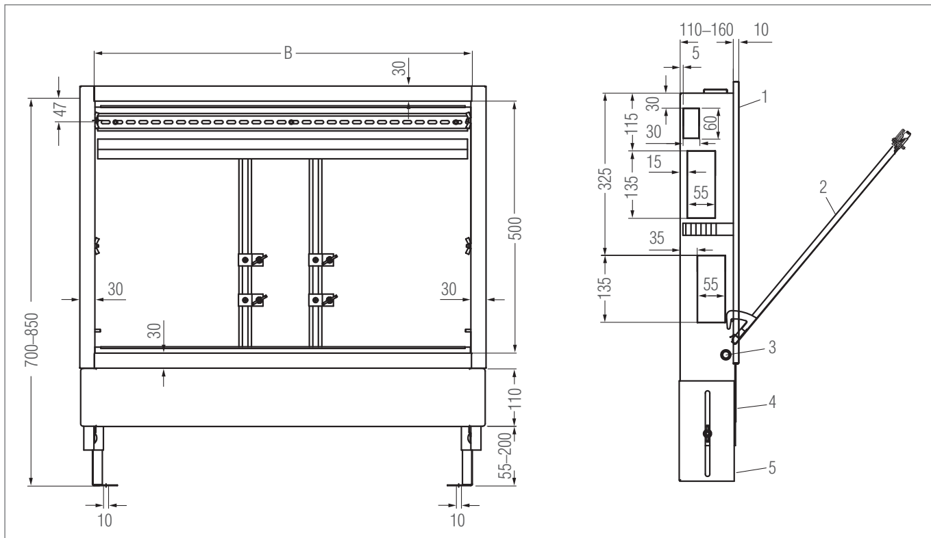
Рис. 6-5 Распределительный шкаф
