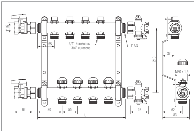
Рис. 6-3 Присоединительные размеры распределительного коллектора НКV
