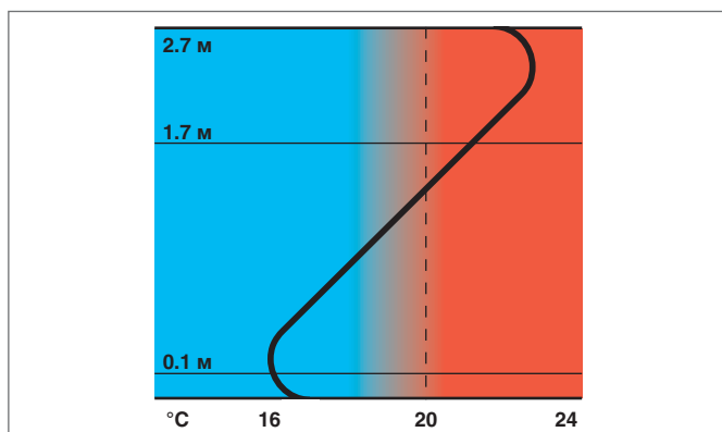
Рис. 2-4 Радиаторное отопление
