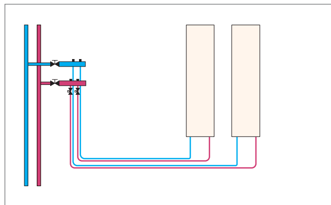
Рис. 4-40 Схема независимого присоединения стеновых панелей обогрева / охлаждения
