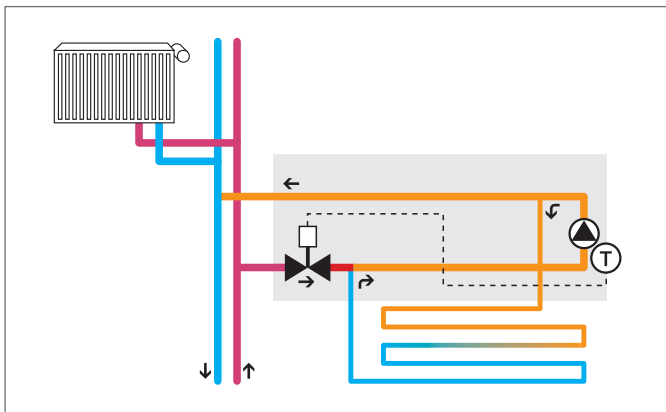
Рис. 7-6 Схема системы
