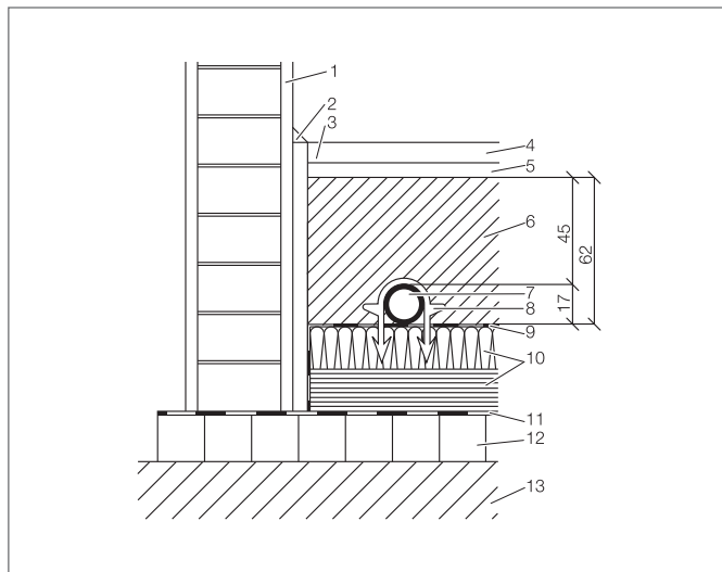
Рис. 3-29 Маты (комбинированная тепло- и шаговзвukoизоляция) с гарпун-скобами для крепления отопительной трубы RAUTHERM S
