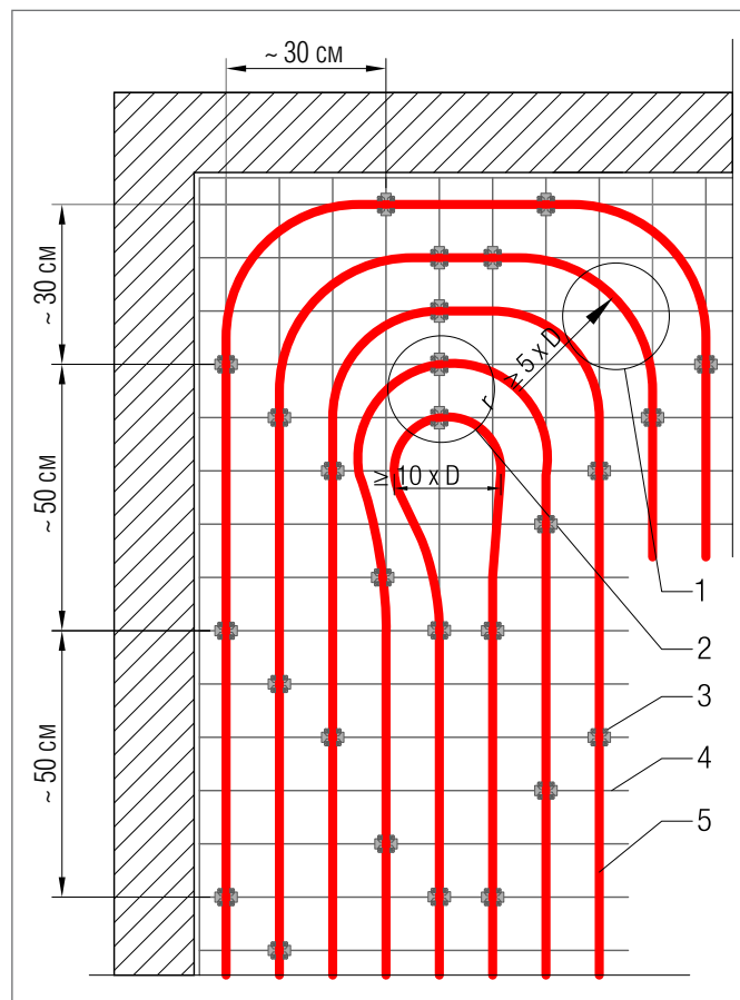
Рис. 3-46 Формирование разворотной петли в регистре отопительных труб. Пример укладки трубы RAUTHERM S 17 x 2,0 с шагом 100 мм на мате RTM 100
