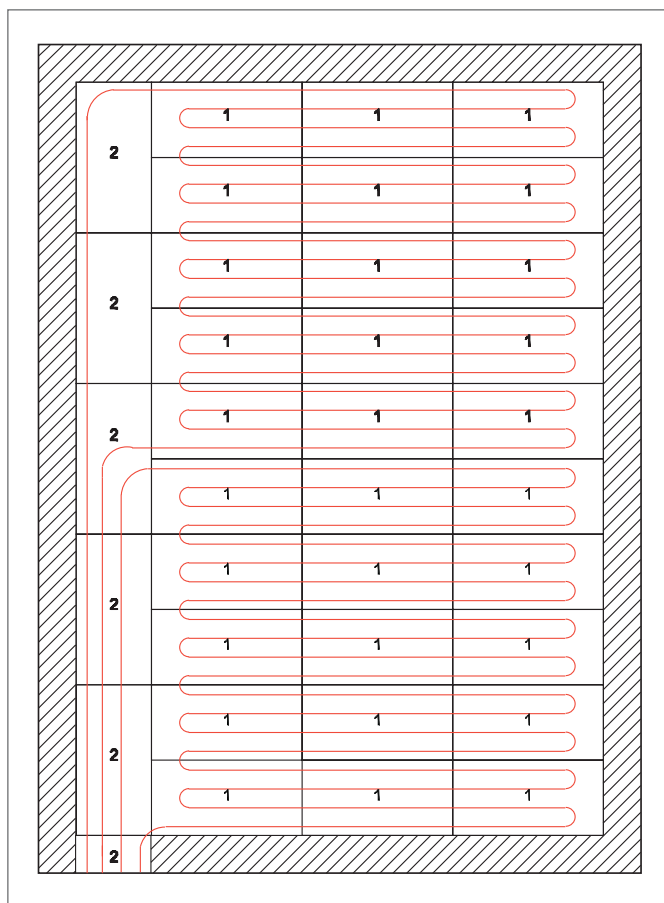
Рис. 3-65 Пример плана укладки труб в теплоизоляционные маты TS-14 1 теплоизоляционные маты TS-14 с закрепленными теплопроводными и поворотными пластинами TS-14 2 дополнительные элементы REHAU
