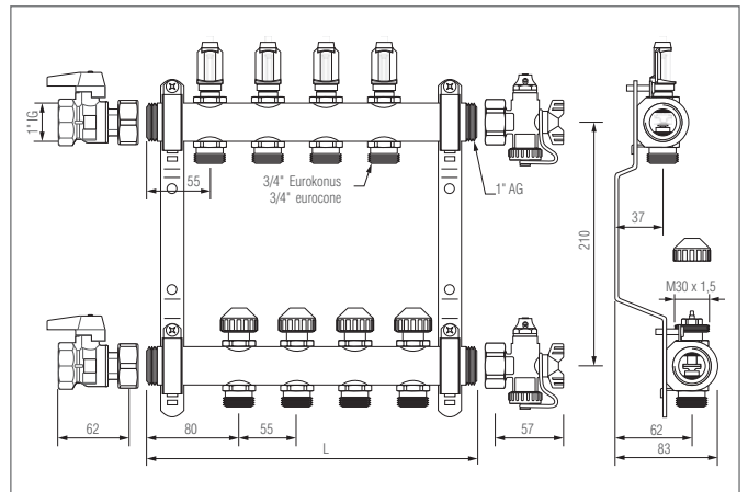
Рис. 6-4 Присоединительные размеры распределительного коллектора НКV-D
