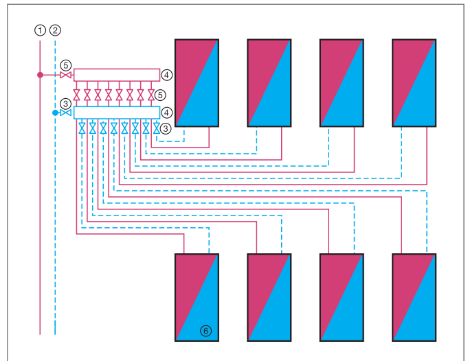
Рис. 8-29 Схема подключения к коллектору
