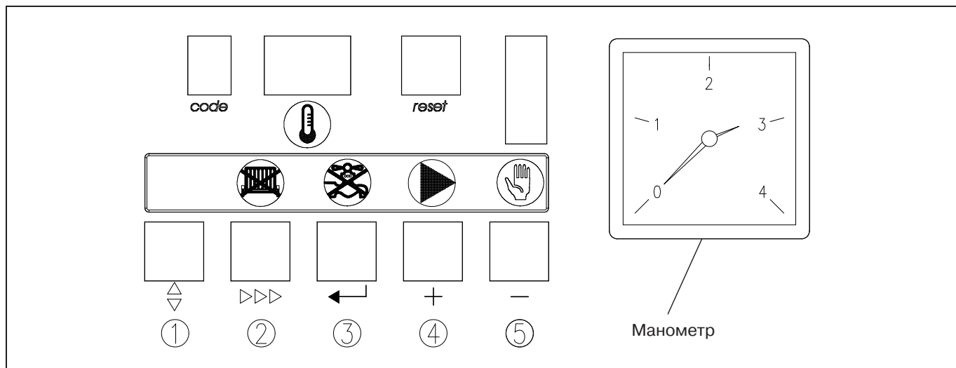
Abb.3: Панель управления
