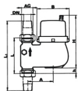
Вертикальный монтаж — резьбовое соединение
