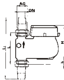
рис. 2 Счетчик воды М-Н (вертикальный монтаж)
