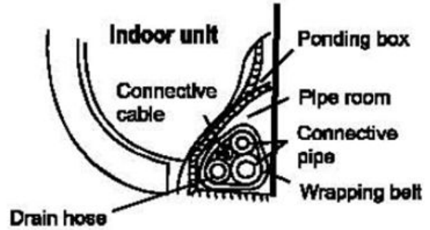
Indoor unit - внутренний блок, connective cable - соединительный кабель, drain hose - дренажный шланг, ponding box - отстойник, pipe room - ниша для труб, connective pipe - соединительные трубы, wrapping belt - обвязка
