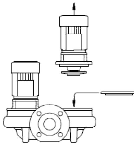
Fig. 4 Applicazione della flangia cieca
