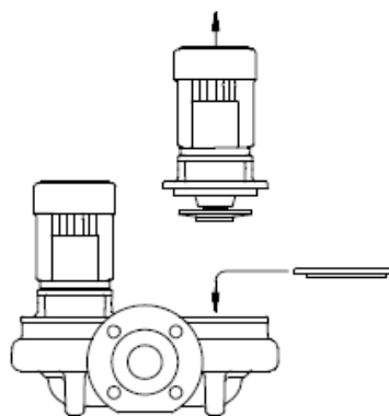
Fig. 4 Montieren der Blindflansche
