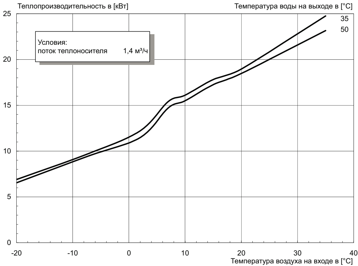
Потребление мощности (вкл. долю мощности насоса)
