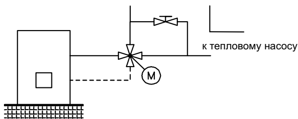
Рис. 8.14: Открытие байпасного клапана для обеспечения максимальной температуры подающего контура
