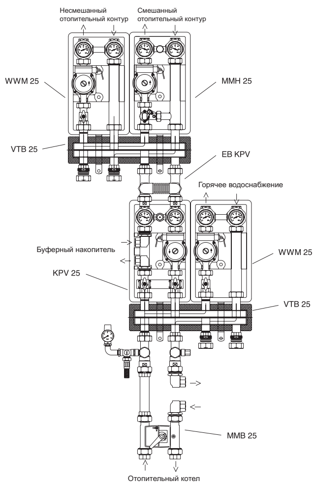
Рис. 8.2: Возможности комбинирования в распределительной системе горячего водоснабжения
