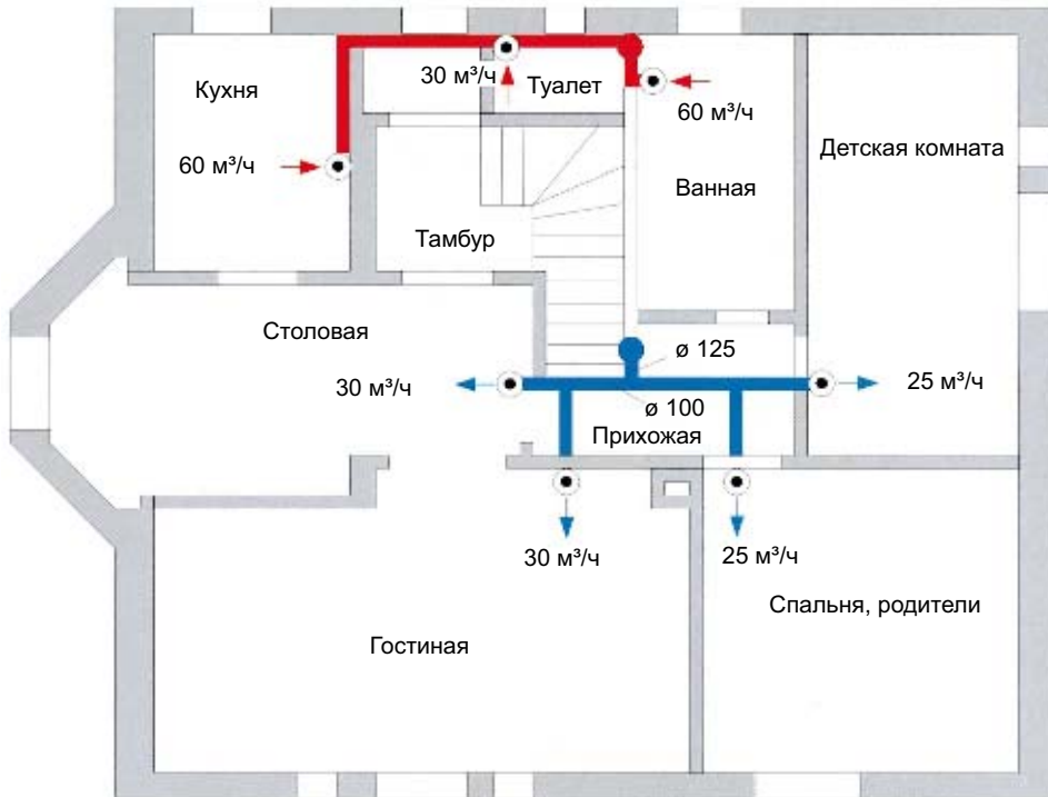
Рис. 6.7: Фрагмент из проекта вентиляционной установки с центральной подачей приточного и отработанного воздуха
