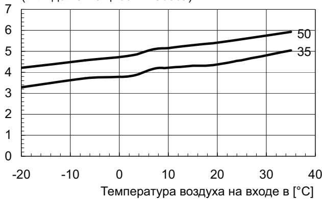
Коэффициент мощности (вкл. долю мощности насоса)
