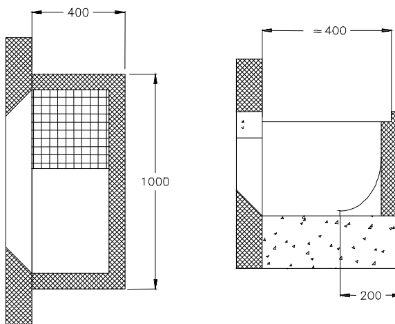
Рис. 2.1: Минимальные размеры световой шахты
