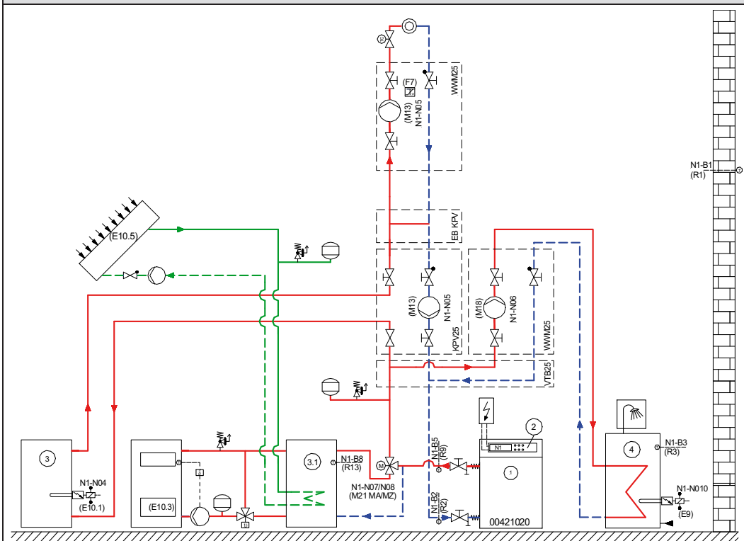
Рис. 8.38: Схема обвязки для бивалентного регенеративного режима работы твердотопливного котла с регенеративным накопителем, одним отопительным контуром с последовательно соединенным буферным накопителем и функцией приготовления горячей воды
