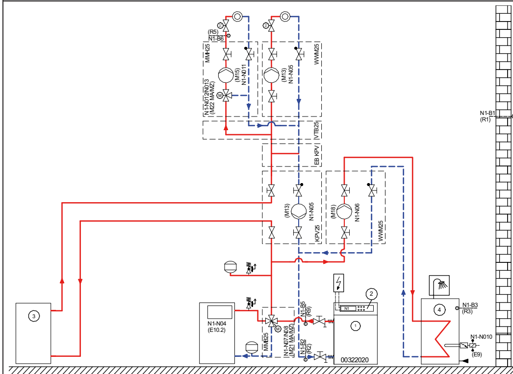
Рис. 8.34: Схема обвязки для бивалентного режима работы теплового насоса с отопительным котлом, двумя отопительными контурами, последовательно соединенным буферным накопителем и функцией приготовления горячей воды.
