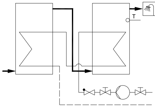
Рис. 6.3: Рядное подключение бойлеров
