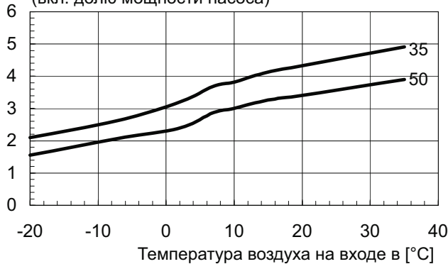
Коэффициент мощности (вкл. долю мощности насоса)
