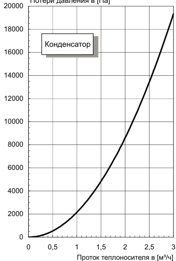
Потери давления в [Па]
