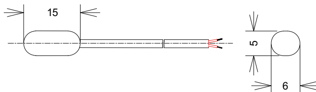
Рис. 7.10: Габариты датчика рециркулирующего потока Norm-NTC-10 в пластмассовом корпусе
