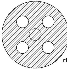
Рис. 3.8: Вид двойного U-образного зонда в разрезе с заполняющей трубой.
