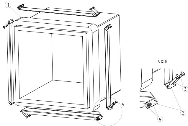
Рис. 2.9: Уплотнительная манжета для воздушных каналов
