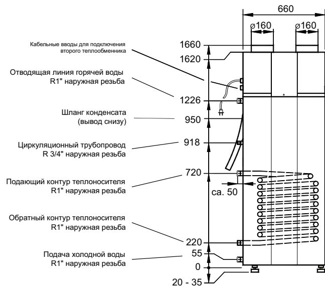
Рис. 6.5: Вводы и размеры теплового насоса горячего водоснабжения BWP 30HLW с расположенным внутри дополнительным теплообменником
