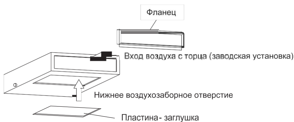
Рис. 10.31 — Установка фланца снизу блока
