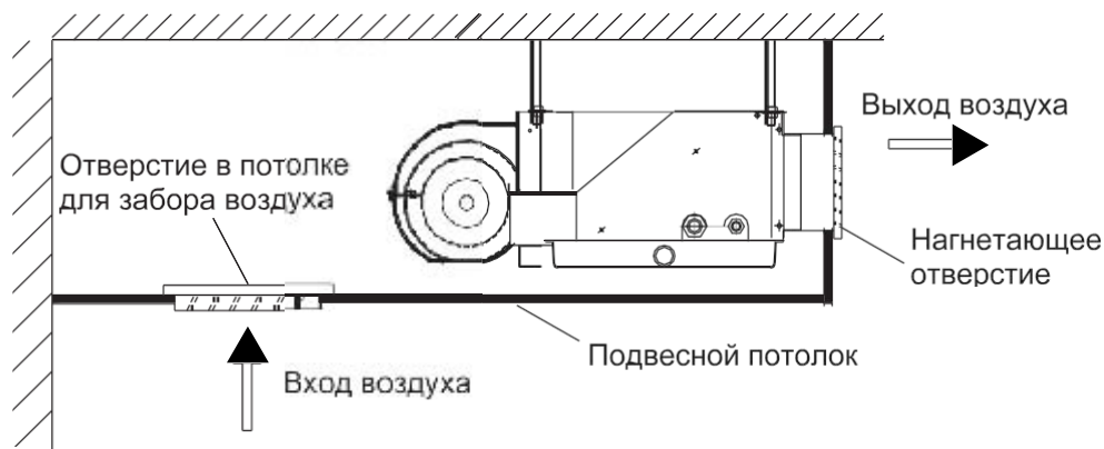
Рис 10.29 — Установка блока без воздуховодов
