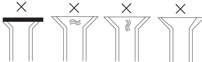
Рис. 11.3 — Примеры неправильной развальцовки
