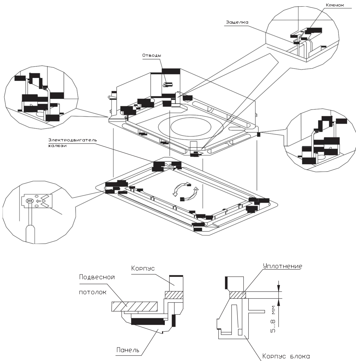
Рис. 10.20 — Установка панели
