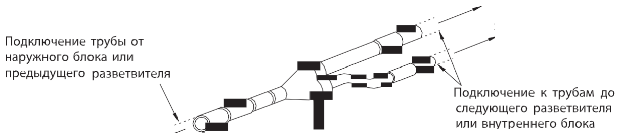
Рис. 11.4 — Подключение разветвителя
