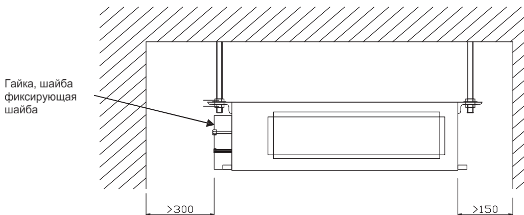
Рис. 10.24 — Размещение блока
