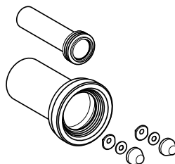
Комплект подсоединения к канализации
