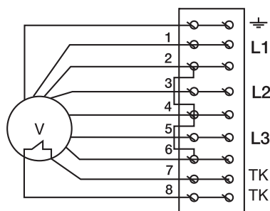
▲-соединение
