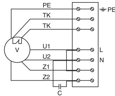
Схема №2 (230 В, 1 фаза)
