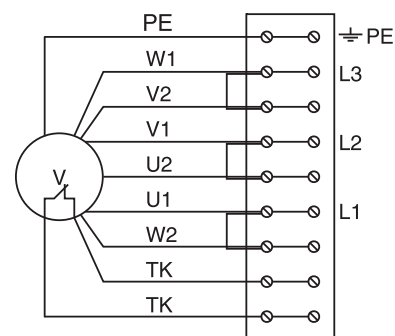
Δ-соединение
