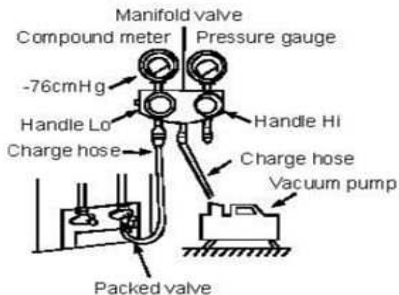
Manifold valve - распределительный клапан, compound meter - индикатор разряжения, pressure gauge - манометр, -76cmHg - -76 см рт. ст., handle Lo - маховичок низкого давления, handle Hi - маховичок высокого давления, charge hose - нагнетательный шланг, vacuum pump - вакуумный насос, packed valve - герметизирующий клапан
