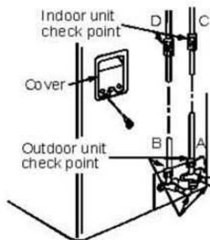
Indoor unit check point - место проверки внутреннего блока, outdoor check point - место проверки наружного блока, cover - крышка
