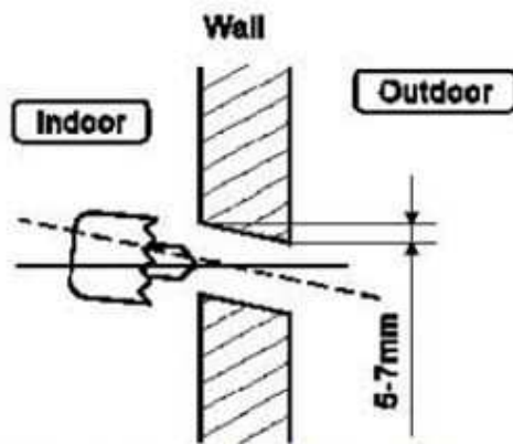
Wall - стена, Indoor - помещение, Outdoor - улица, 6-7 mm - 6-7 мм
