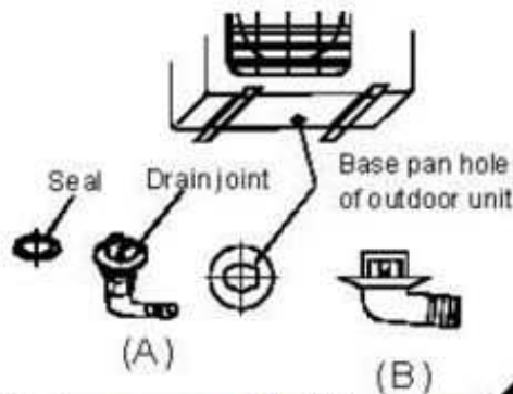
Seal - уплотнение, drain joint - дренажная муфта, base pan hole of outdoor unit - главное отверстие лотка наружного блока
